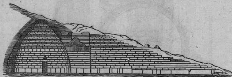
Fig. 4. a — Sepultura de Mycenas (Thesouro de Atreu) — Côte
