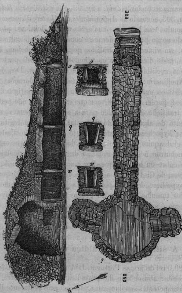
Fig. 6.ª — Sepultura de Alcalar (Algarve)
